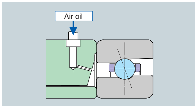
Fig. 9.23 HSF type
