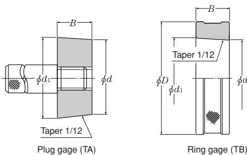
Fig. 6.29 Taper gage
