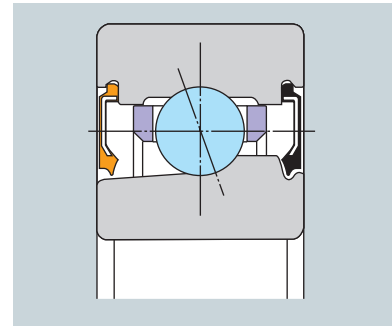
Fig. 9.37 BNS LLB type
